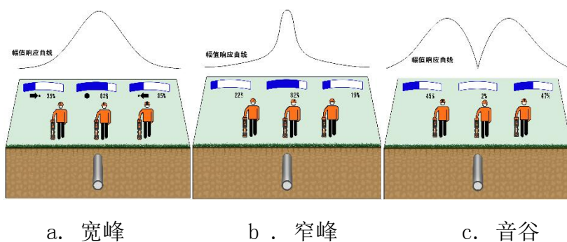
图 6- 1 不同模式下的信号响应
