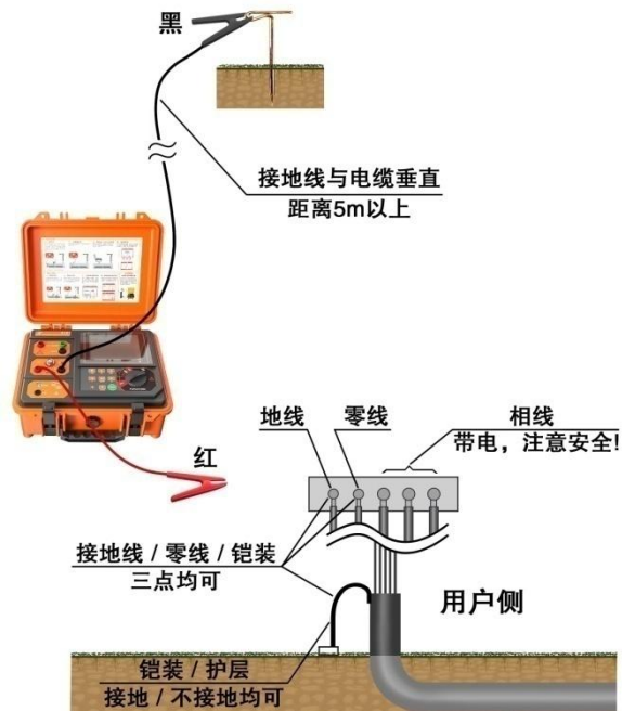
图 5- 21 运行电缆零线 / 地线 / 护层注入法
