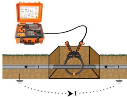
图 5- 15 卡钳耦合接线图
