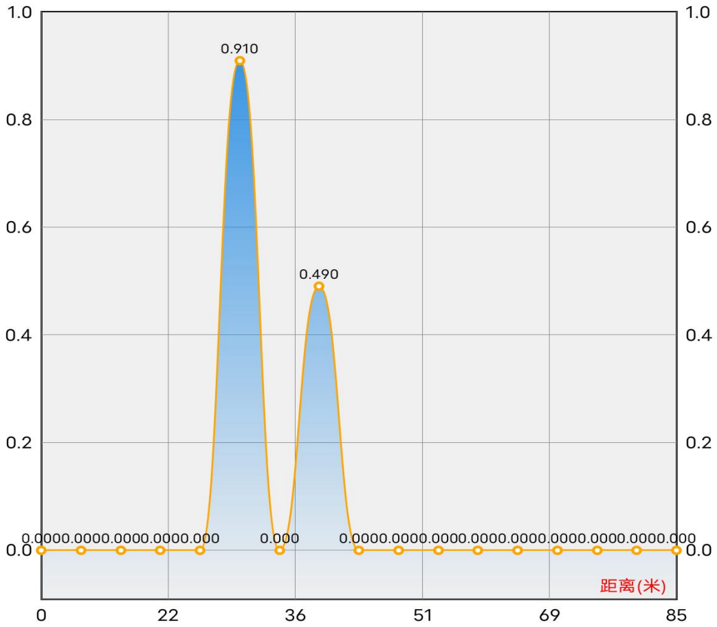
图 7-8 深度变化曲线图
