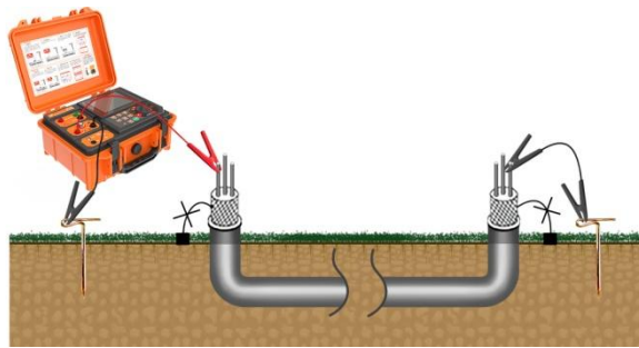
图 5- 4 芯线-大地接法接线图
