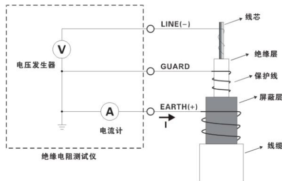
图 8- 9 屏蔽端 GUARD 线使用示意图
