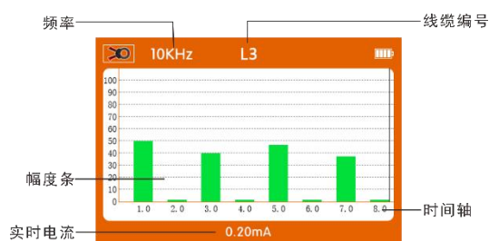
图 6- 21 10kHz 以上的线缆识别界面
