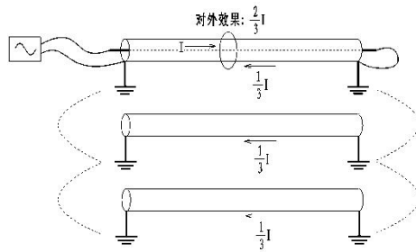
图 5- 10 并行电缆的分流效果
