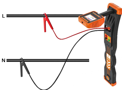
图 8- 11 电压测量接线图
