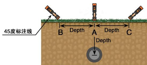
图 6- 13 音谷 45^\circ 法测深
