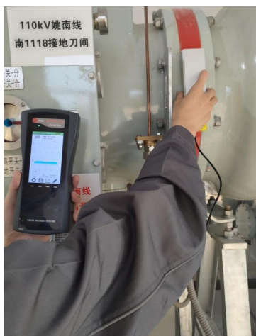
特高频传感器用法
