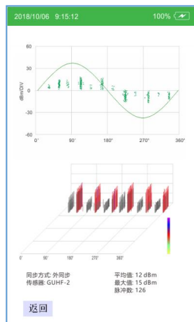
自由金属颗粒放电
