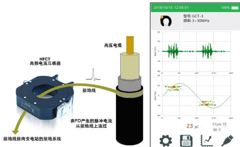
HFCT 接线方式
