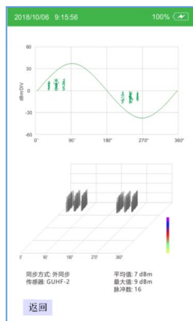
悬浮电位体放电
