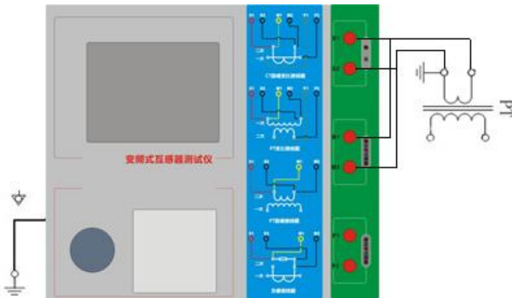
图 2.7 PT 直阻、励磁试验接线方式
