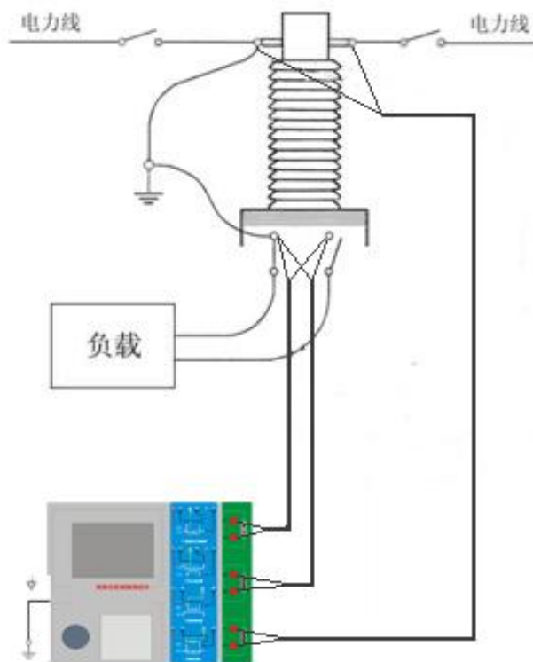
图 C.1 典型接线方式
