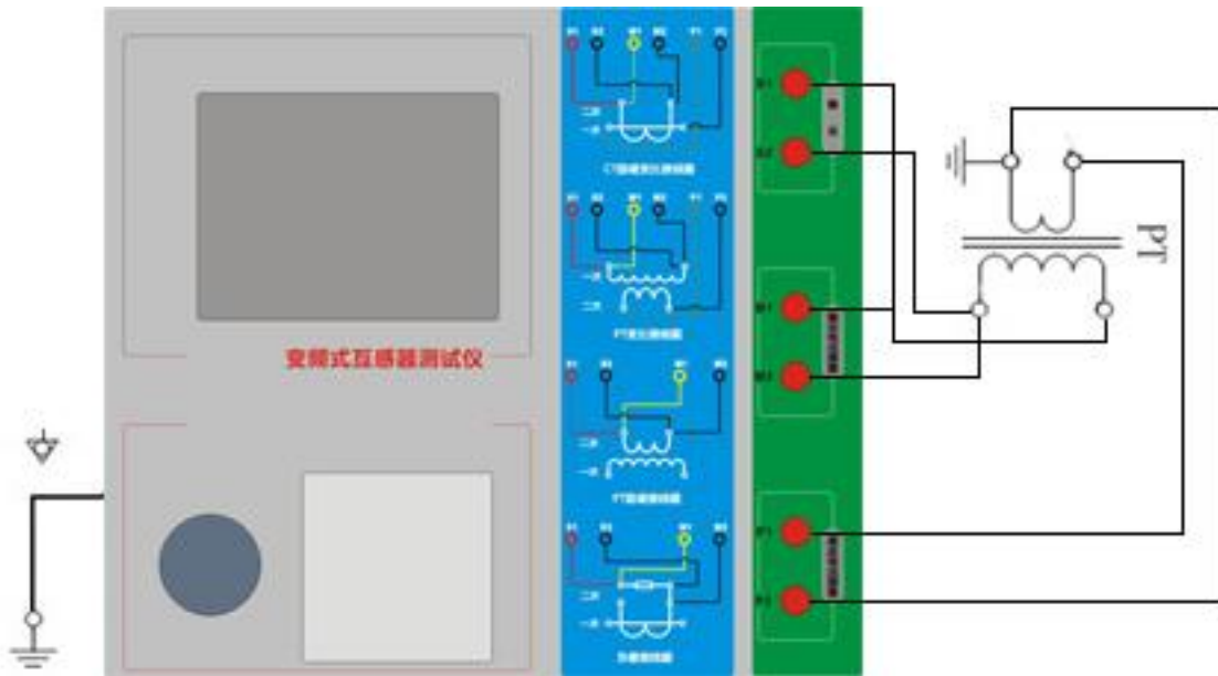
图 2.8 PT 变比、极性试验接线方式
