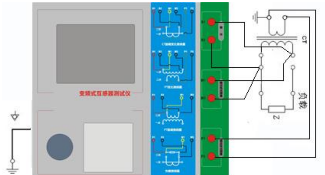
图 2.1 CT 直阻、励磁、变比试验接线方式
